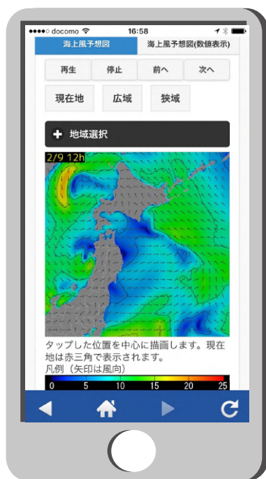
海上風予想図
