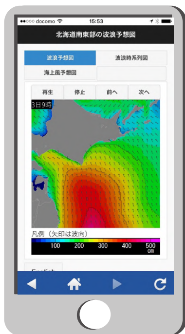
波浪予想図
