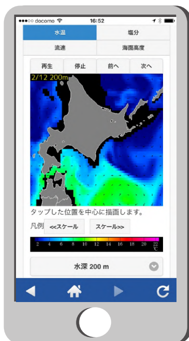
水温予想図
